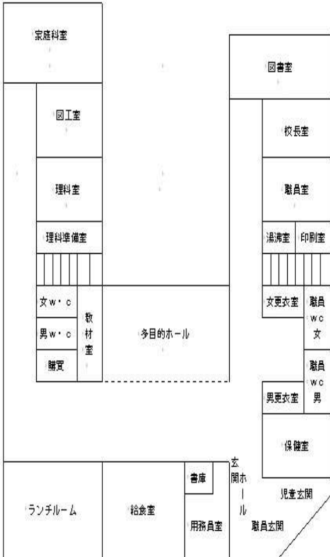
1階
